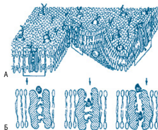
Мал 2. Тривимірна рідинно-мозаїчна модель клітинної мембрани (за Сінгером-Ніколсоном). А – подвійна фосфоліпідна оболонка, в яку занурені білки; Б – різні етапи руху Na + через клітинну мембрану.
